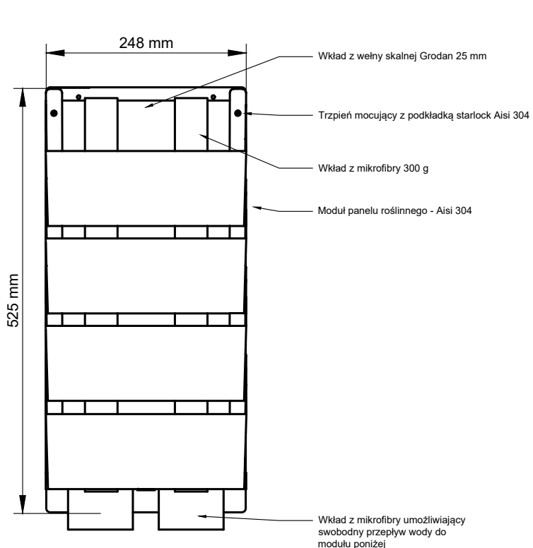
WIDOK - PRZÓD MODUŁU
