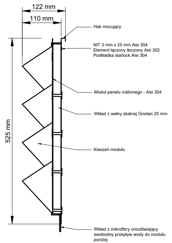
WIDOK - BOK MODUŁU
