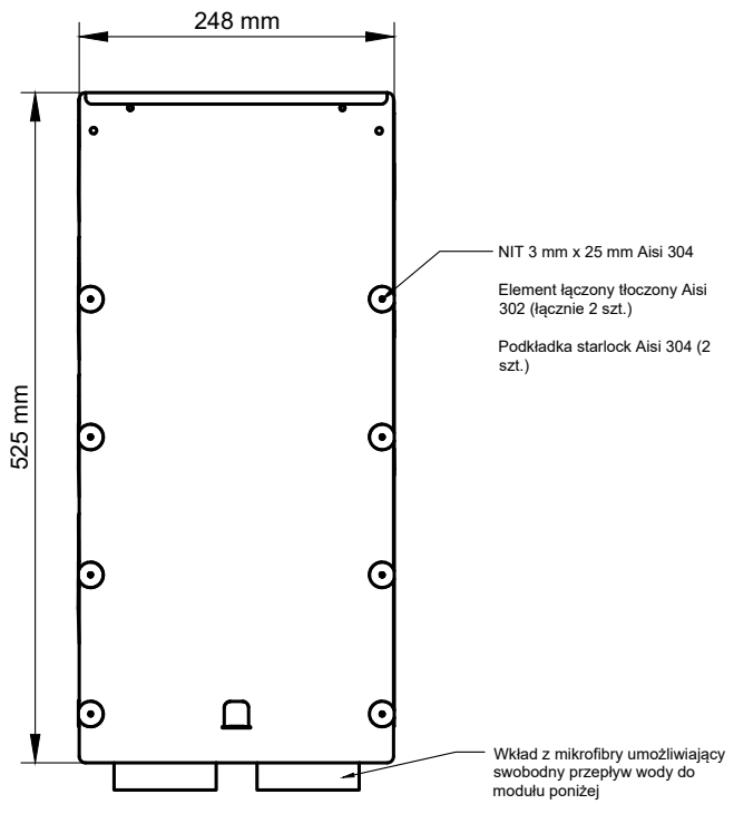
WIDOK - TYŁ MODUŁU
