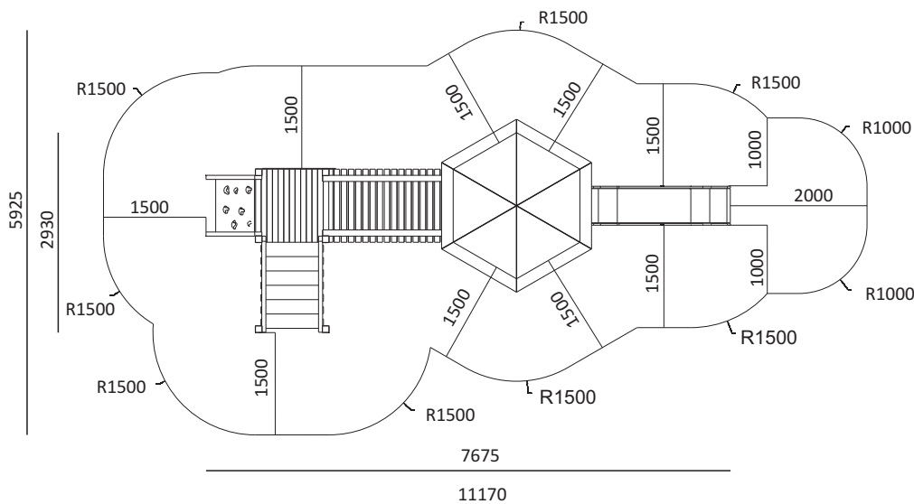
rzut poziomy ze strefą bezpieczeństwa skala 1:100
