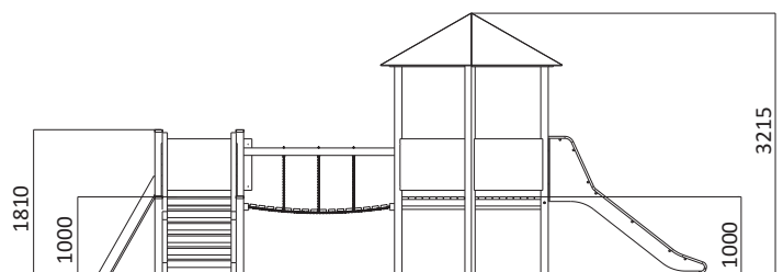
rzut pionowy
