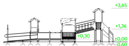
Widok urządzenia
