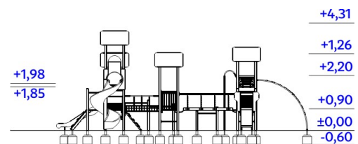
Widok urządzenia
