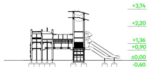
Widok urządzenia
