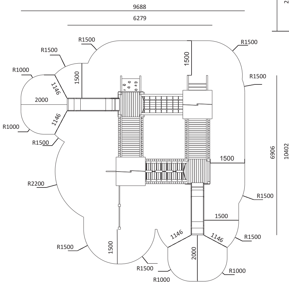
rzut poziomy ze strefą bezpieczeństwa skala 1:100
