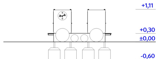
Widok urządzenia
