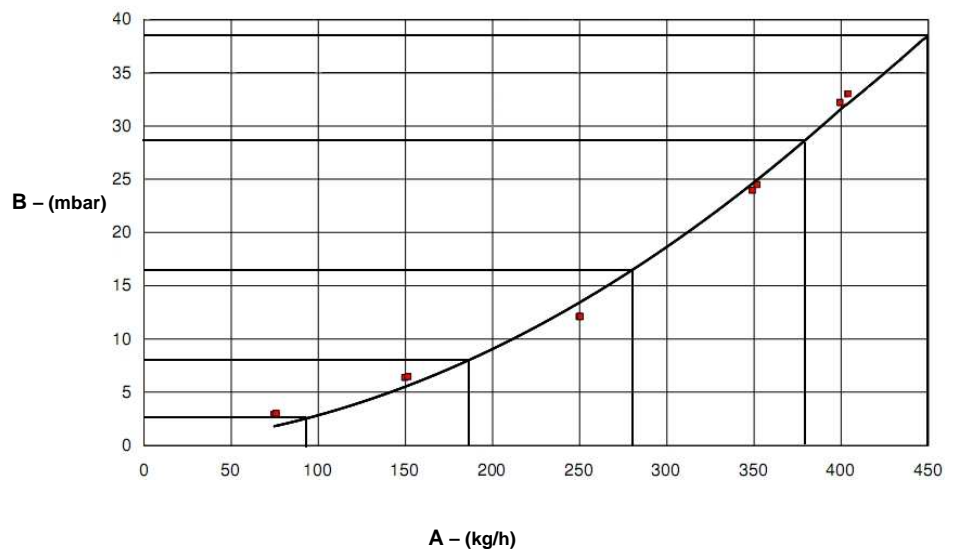
Wykres strat ciśnienia Pressure loss chart / Diagramm Druckverlust
