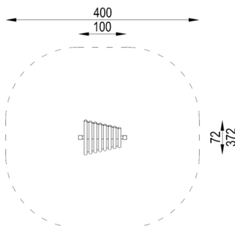
Widok urządzenia
