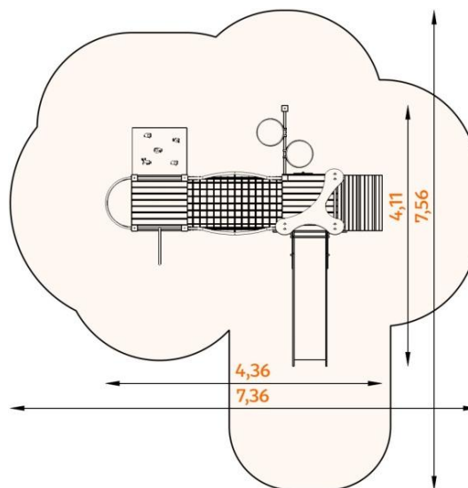
Rzut urządzenia wraz ze strefą funkcjonalną
