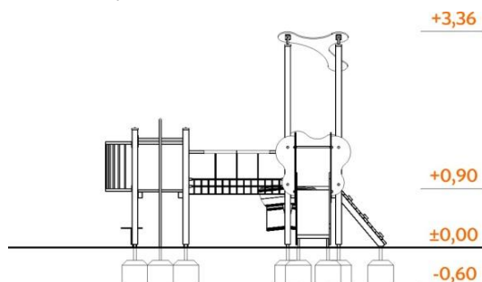
Widok urządzenia
