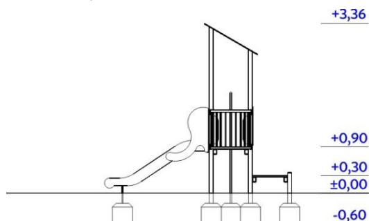
Widok urządzenia
