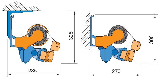
Montaż do sufitu
