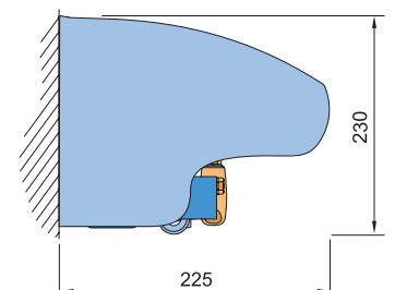
Montaż do ściany (wersja z daszkiem)
