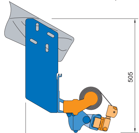
Montaż do sufitu
