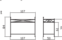
Beauty Schminktisch/ table de-maquillage / dressing table Eisen teilmassiv schmiedeisenfarbig/Glas Fer partiellement massif teinté fer forgé/verre Partial solid iron wrought ironcoloured/glass
